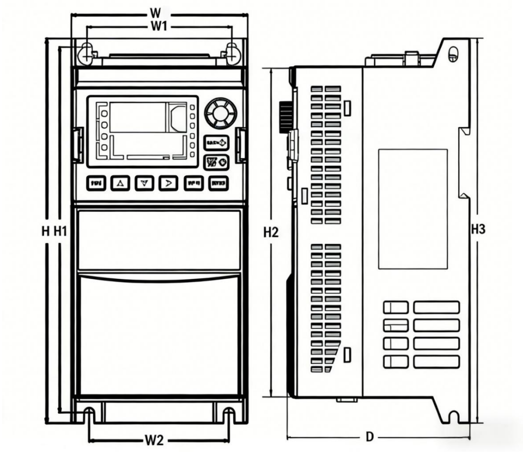
图 1 变频器安装尺寸示意图
