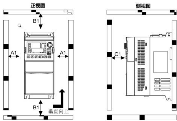
单台机器（T1-T5）安装空间
