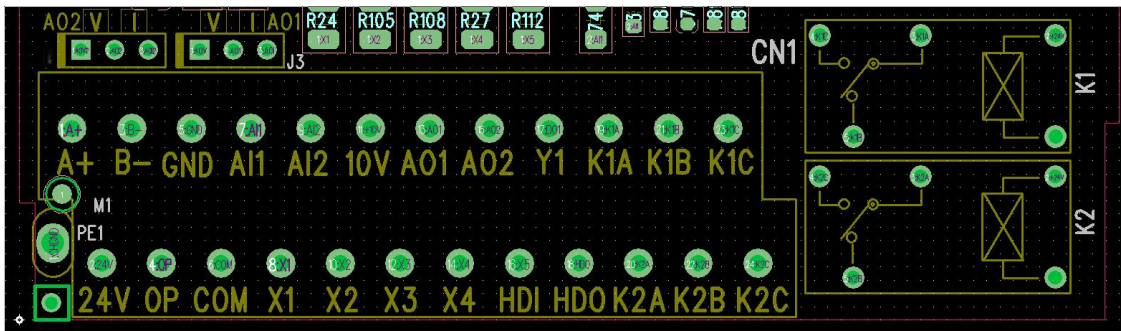
（端子布置图）
