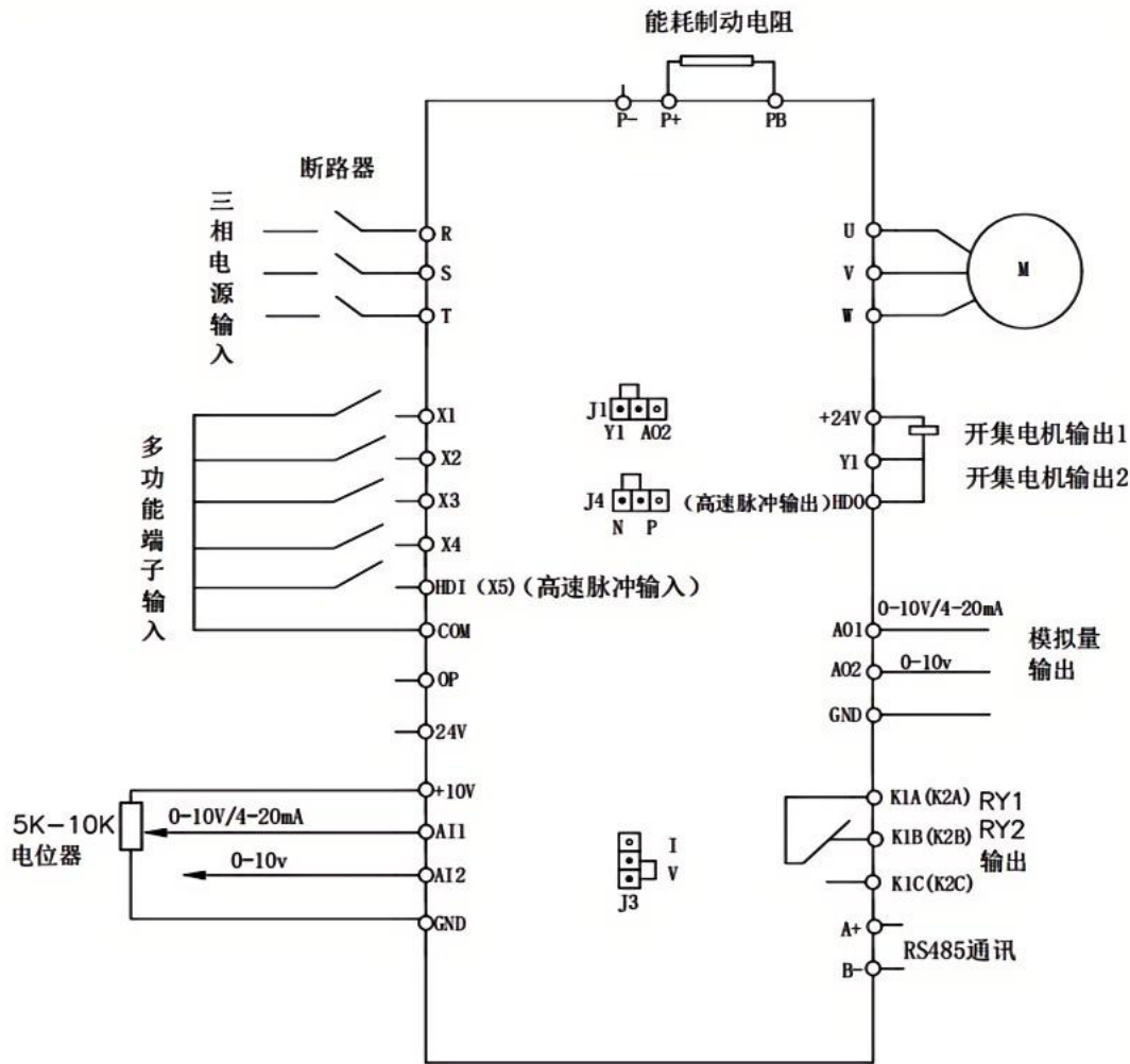
图 2-2 变频器控制回路接线方式
