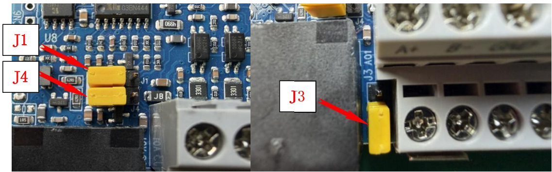
（跳线布置图）
